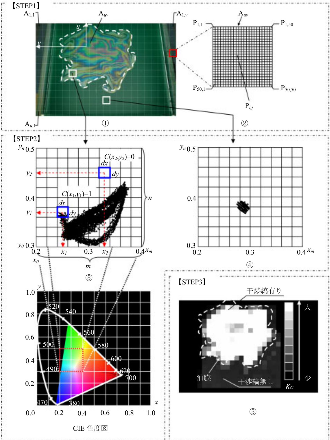
図7 油膜検知処理の流れ(画像の処理過程)
