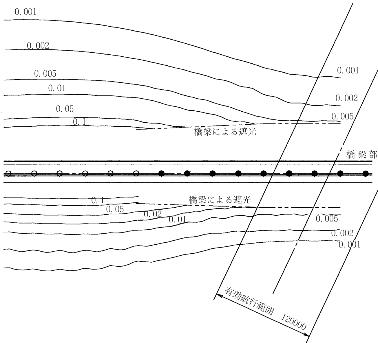
図7 海上面漏れ光 (初期) 照度分布図
