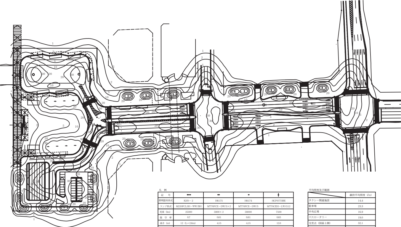
図9 南口中央広場、道路照明、歩道照明、照度分布図
