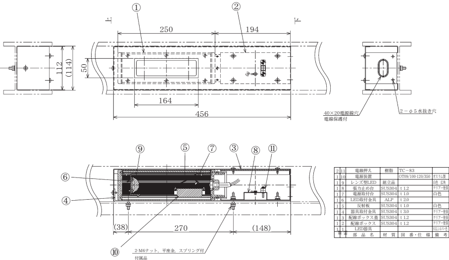
図10 LED アプローチライト寸法・構造図
