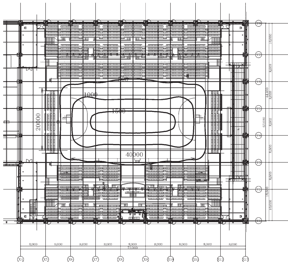
図2 メインアリーナ照度分布図
