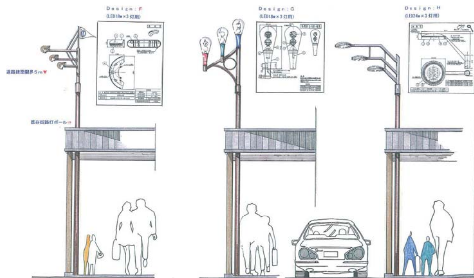
图 4 Design F~H
