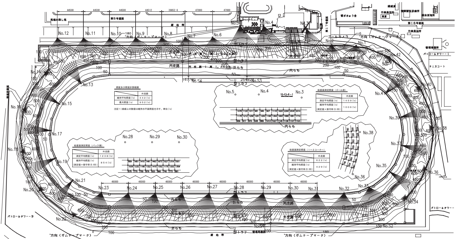
図9 走路照度分布 (鉛直面照度測定結果記入)
