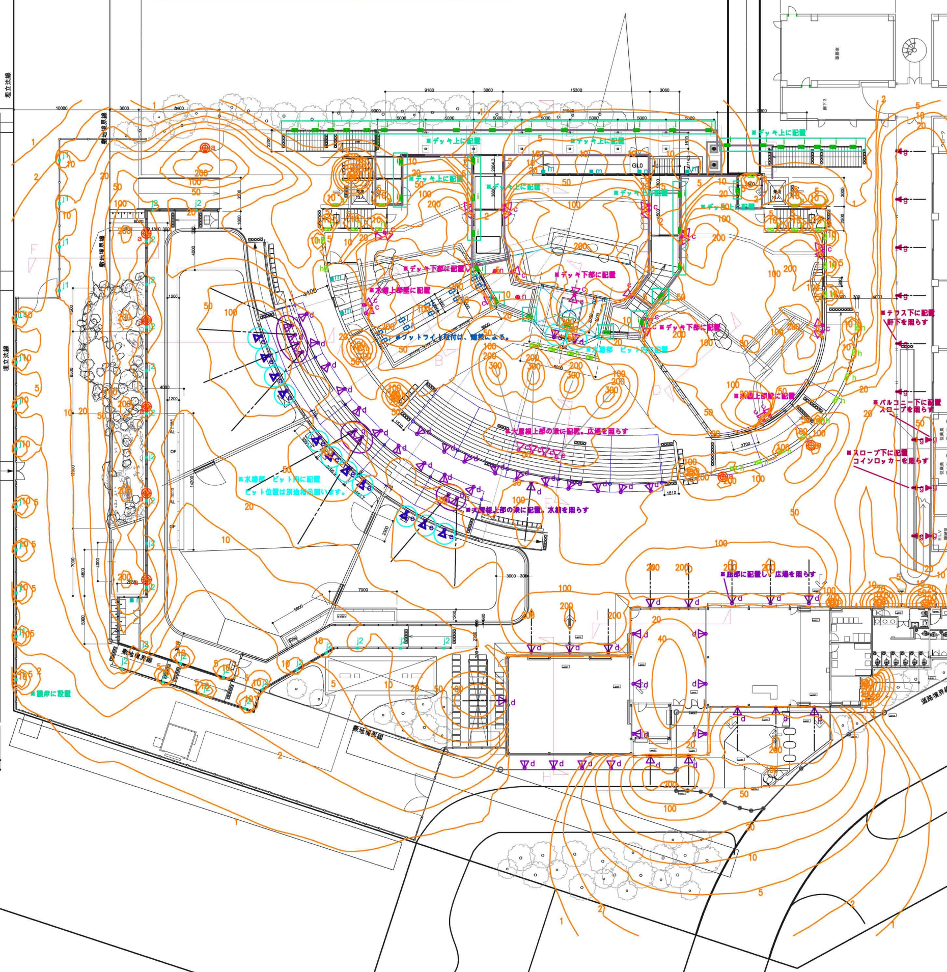
維持照度分布図 A1:S=1/200 A3:1/400
