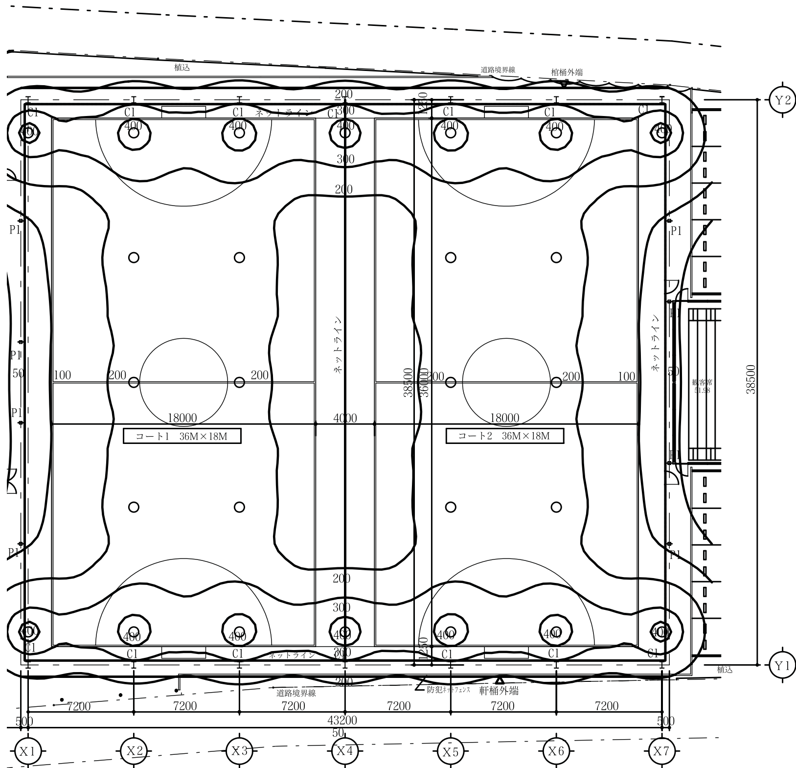
図7 照明設備配置図および照度分布図
