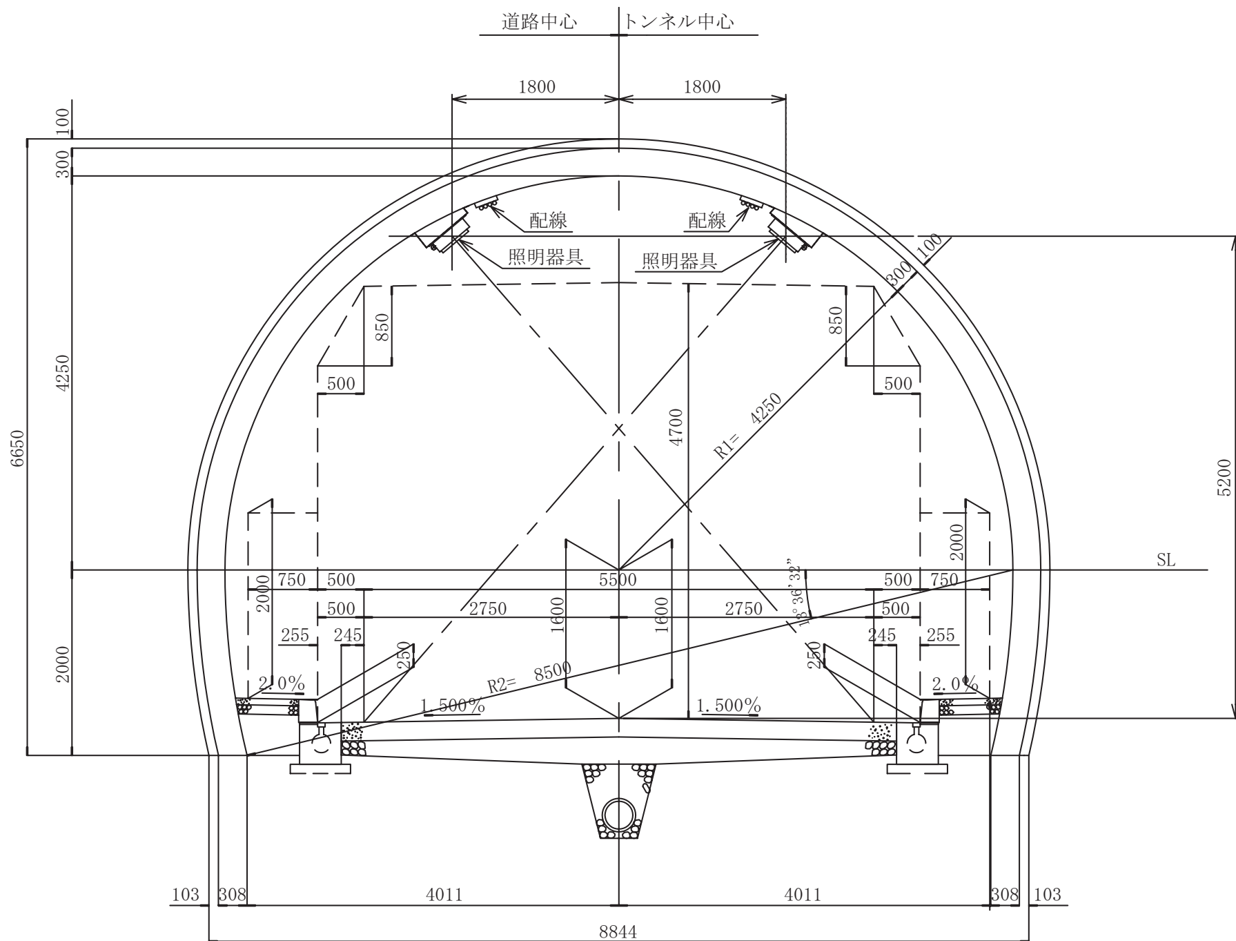
図4 トンネル断面形状
