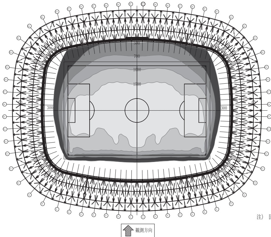
図4 照度分布図 (Jリーグパターン): 鉛直面照度
