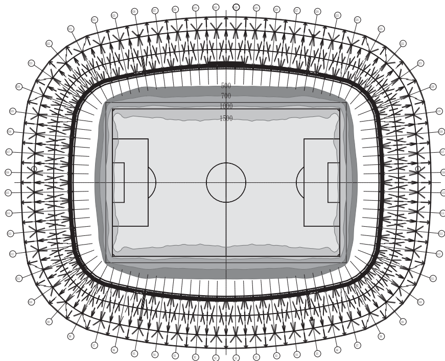
図3 照度分布図 (Jリーグパターン): 水平面照度
