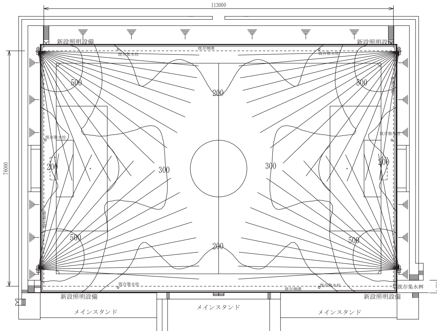
図4 第二球技場水平面照度分布図 (全点灯時, 維持照度)
