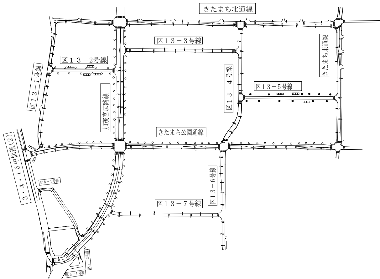
図1 全体計画図
