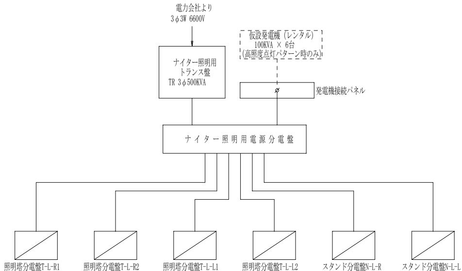
図8 電源系統図
