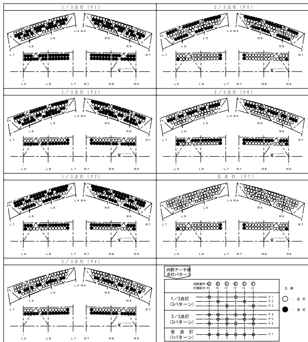
図7 点灯パターン図 (内野アーチ部)
