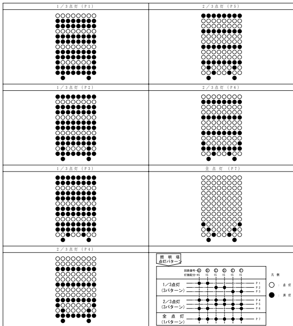
図6 点灯パターン図 (照明塔)
