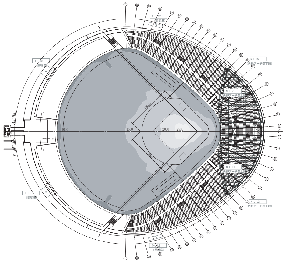
図5 照度分布図 (全点灯時)
