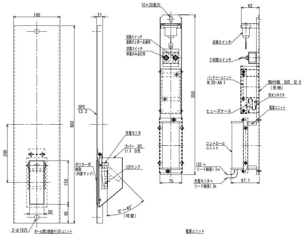
図6 屋外形アイクラクナイン®の外形図
