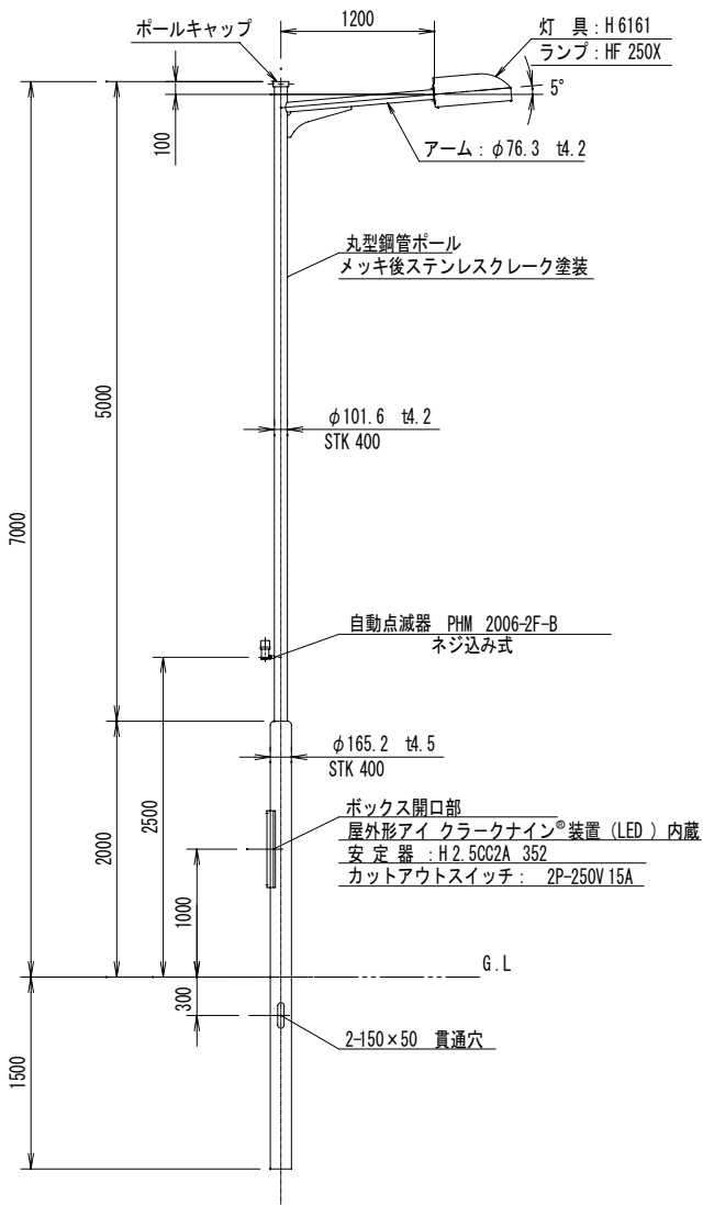
図3 照明灯の外形図
