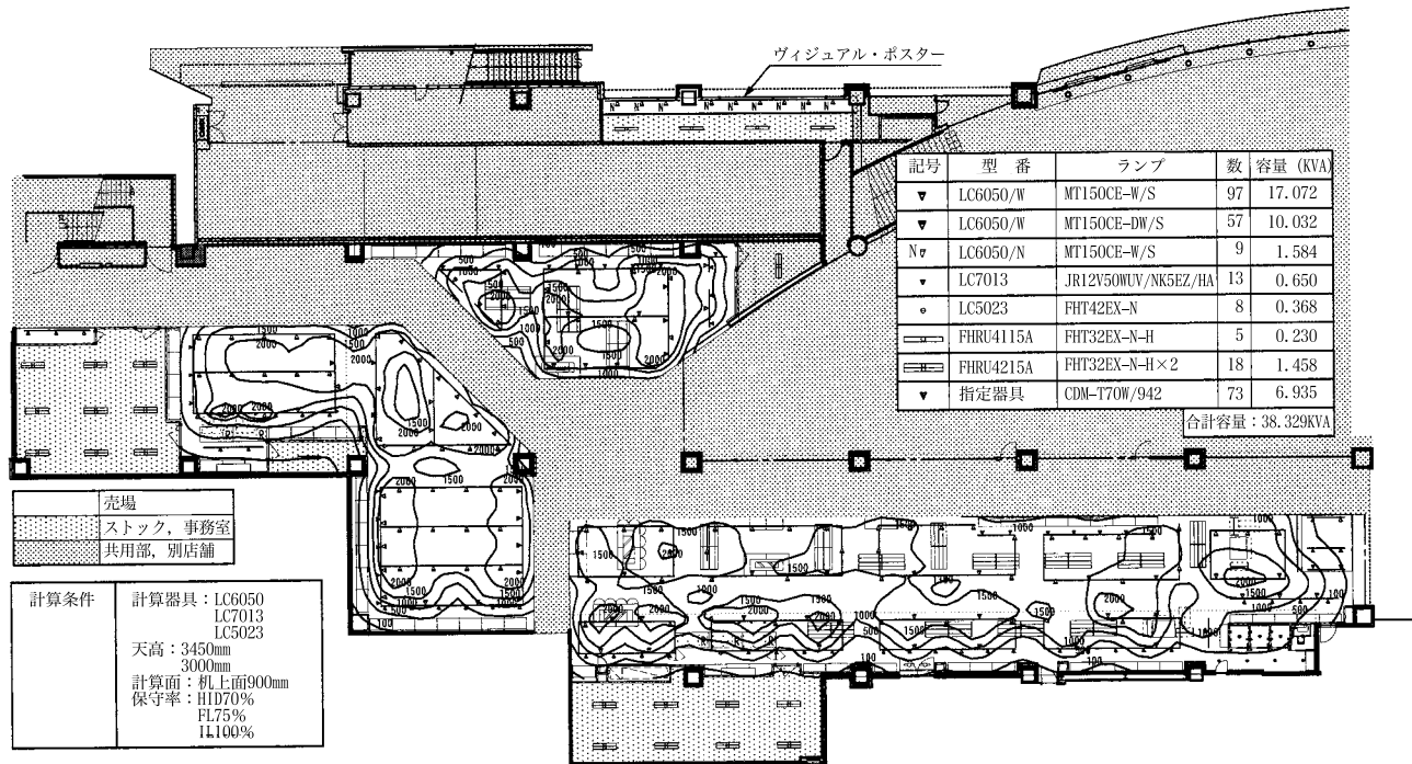
図6 みなとみらい店 照度分布図
