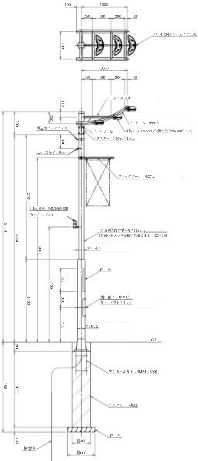
図6 街路灯図面
