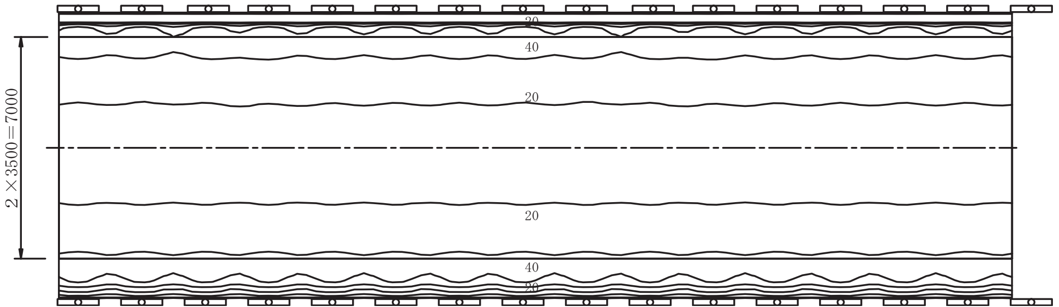
図7 高欄照明部照度分布図
