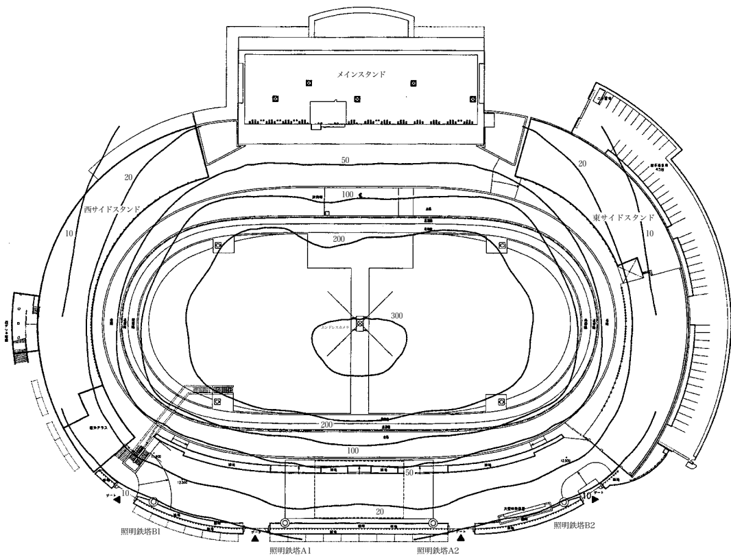
図6 水平面照度分布図（スポーツ1：維持照度）
