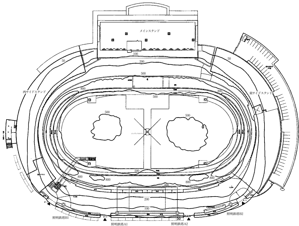
図4 水平面照度分布図（自転車競技1：維持照度）
